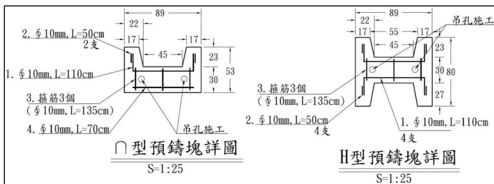
圖 6 H 型塊各部尺寸圖
