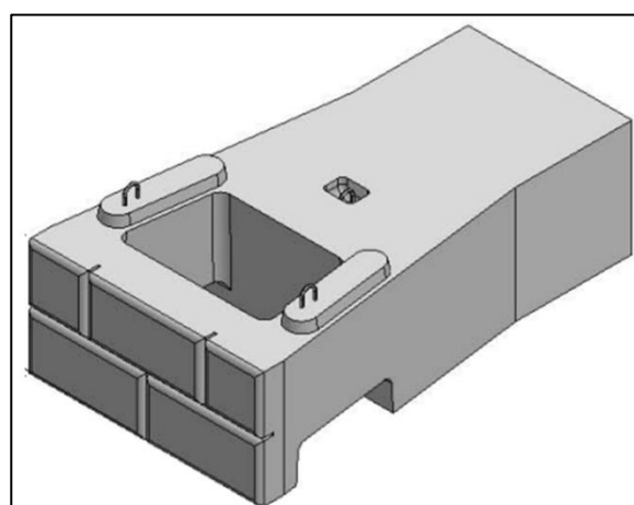
(b)凹凸槽(子母扣)嵌鎖
