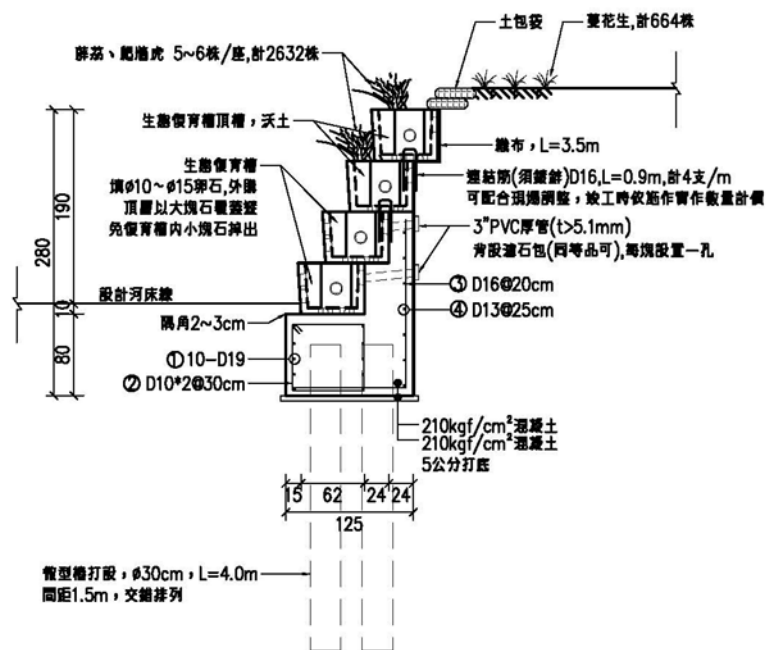
新設生態槽含基礎(H=2.8m) 詳圖
