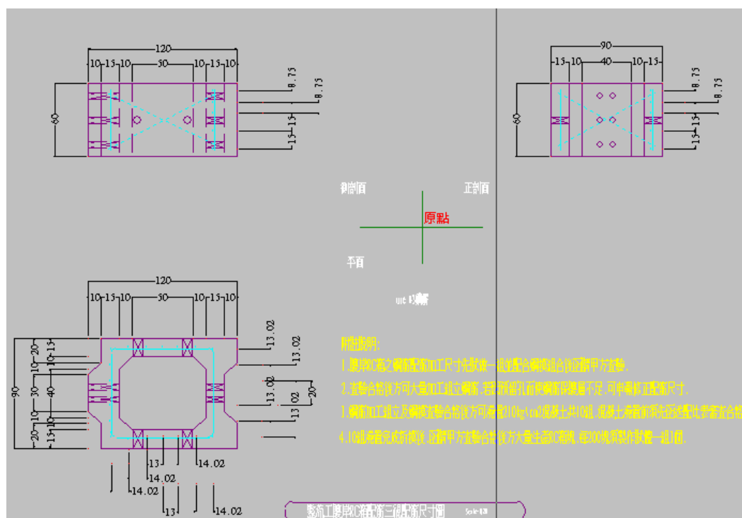
圖 9 RC 箱塊各部尺寸圖
