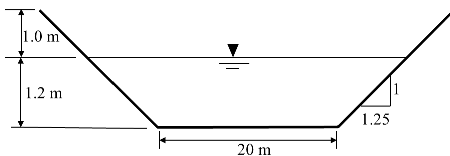
圖 5-2 溪流斷面尺寸圖
