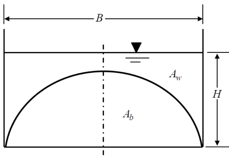
圖 4-5 斷面劃分示意圖
